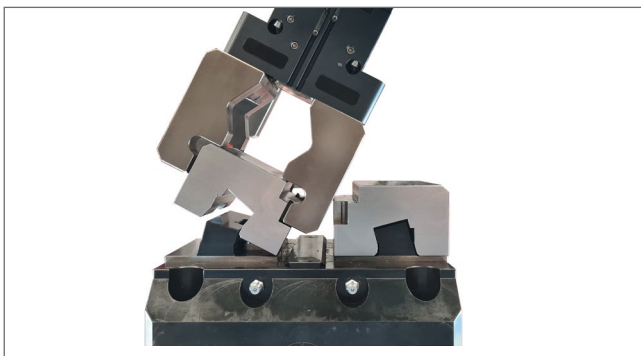
Optionale Spanntechnik: Intelligenter Schraubstock mit automatisch wechselbaren Klickbacken
